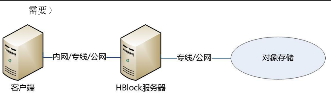
图1. 单机版网络拓扑图
